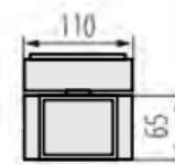
Вид сверху
