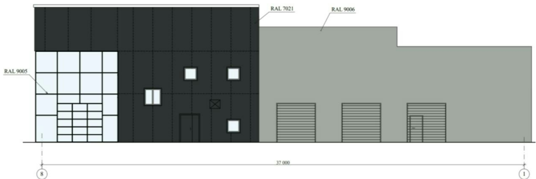
Фасад А - Ж
