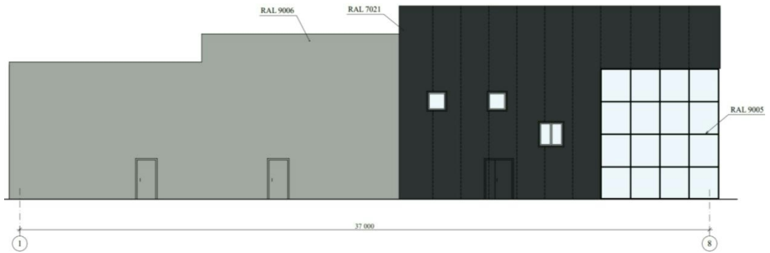
Фасад в осях 8 - 1
