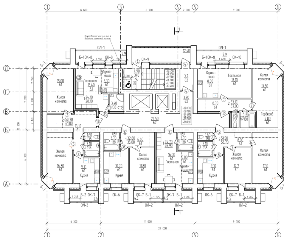
План 7-12 этажей
