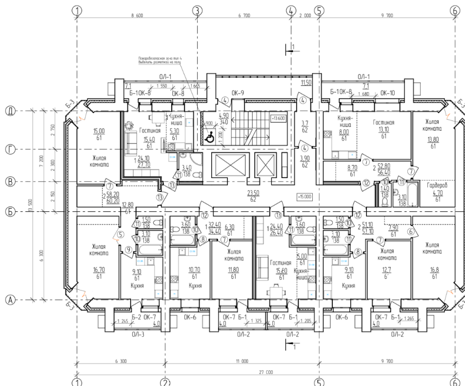
План 7-12 этажей
