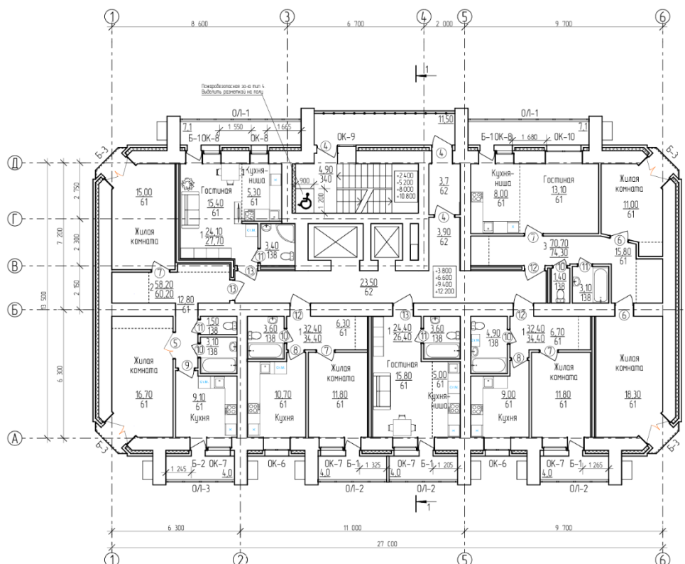
План 2-5 этажей
