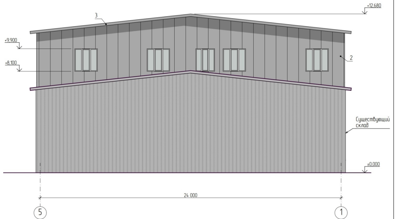
Фасад в осях 5-1
