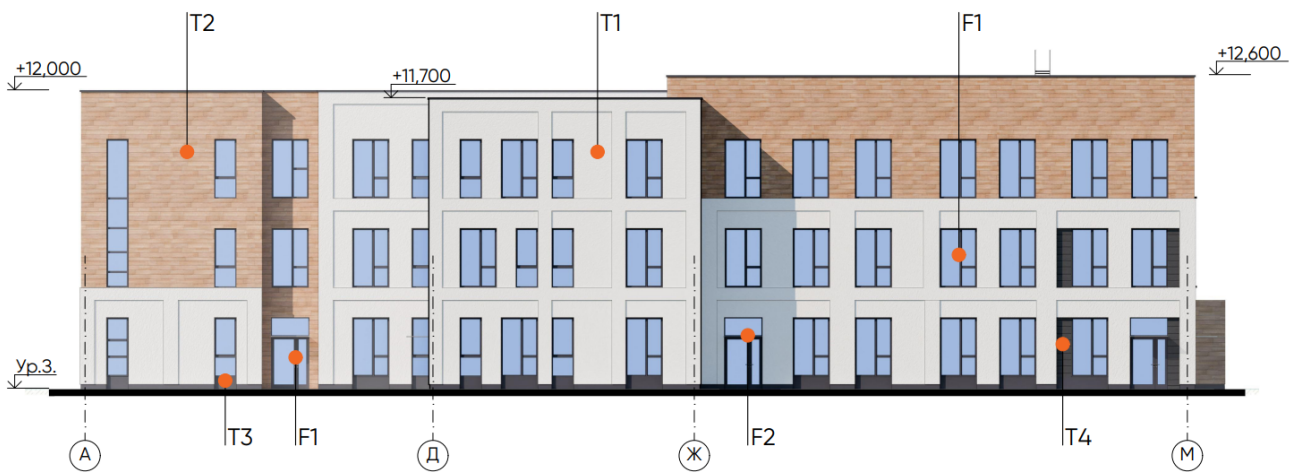
ФАСАД А-М
